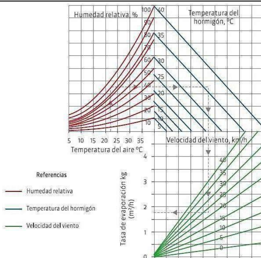
Figura 5-1 - Nomograma para predecir la posibilidad de fisuración plástica.
