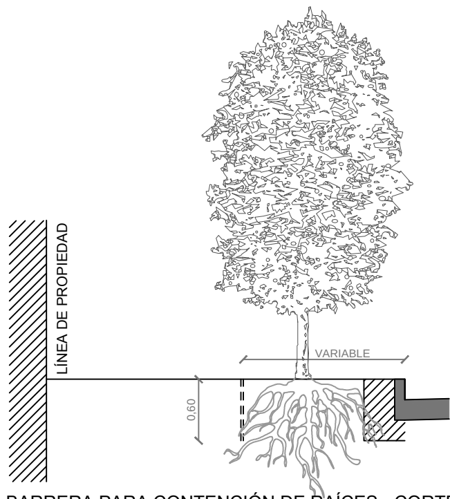
BARRERA PARA CONTENCIÓN DE RAÍCES - CORTE
