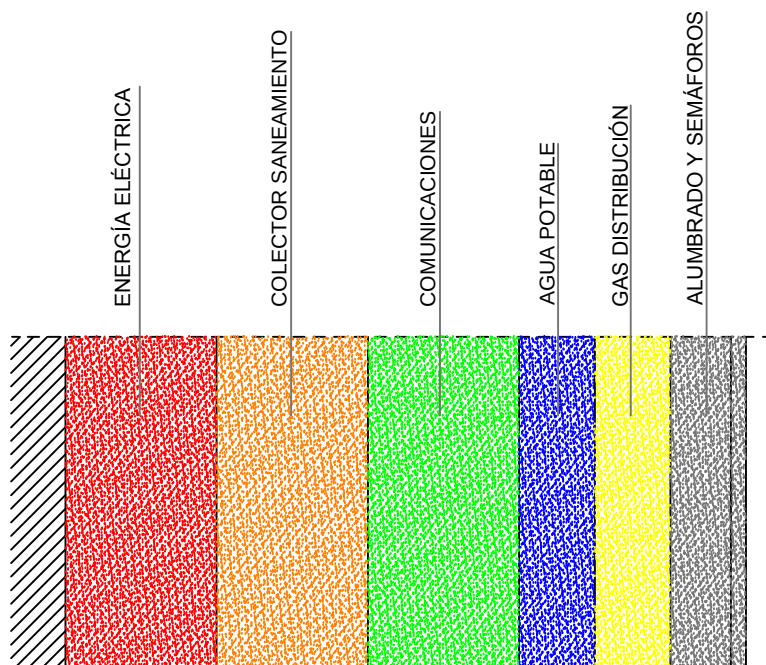
DISPOSICIÓN EN PLANTA DE LAS CANALIZACIONES
